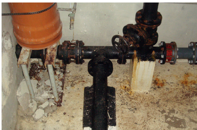
Fig.3: Fuktskader
